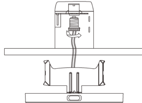
5" / 6" Retrofit
